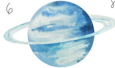
Uranus
